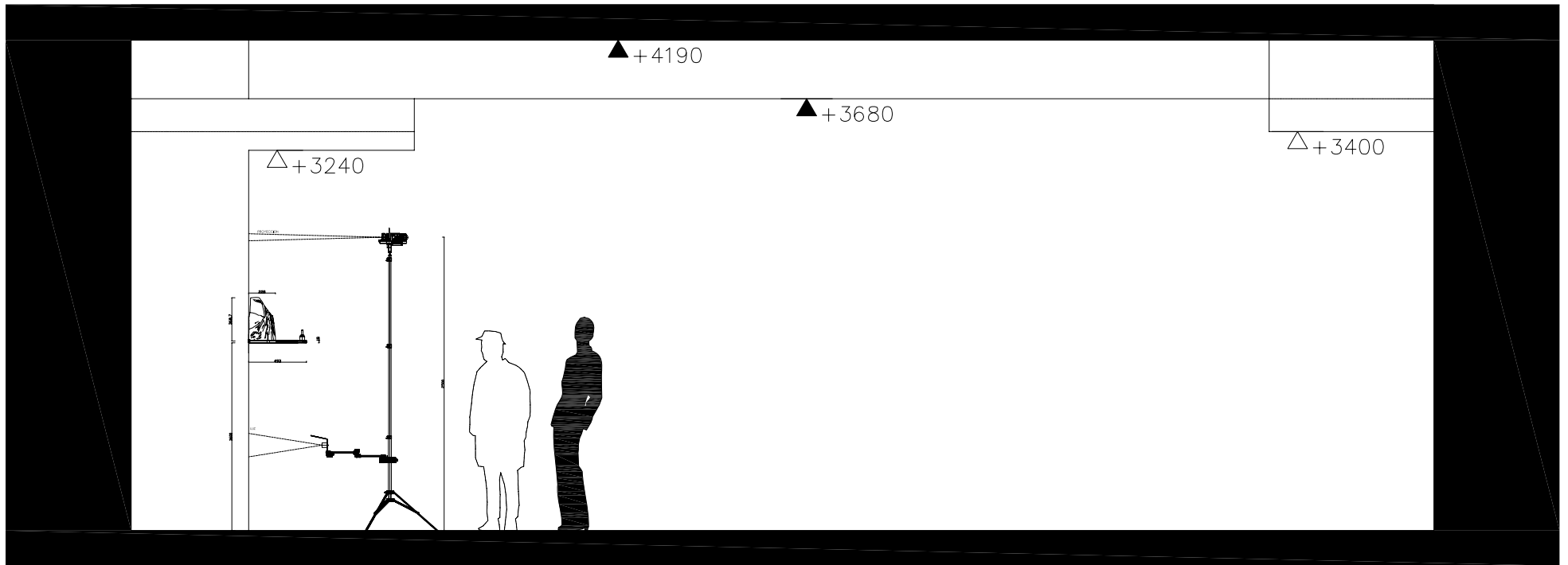
ELEVACION MODULO QUADRIVIUM (unidades en milímetros)
